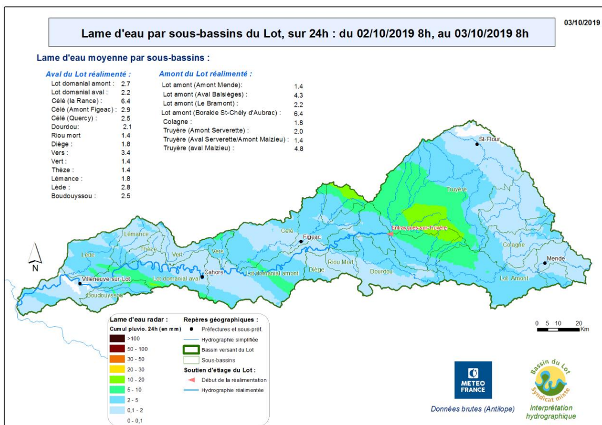
Lame d'eau radar du cumul pluviométrique sur 24 h du 2 au 3 octobre 2019
