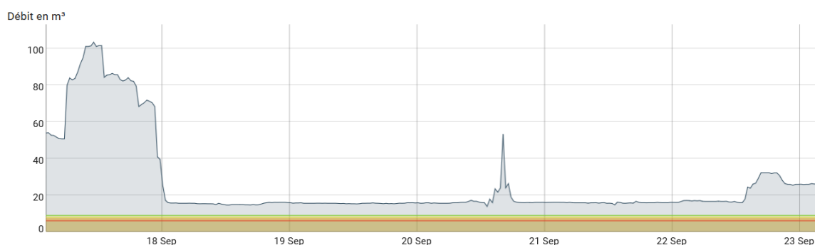
Graphique des débits instantanés enregistrés à Entraygues-sur-Truyère du 17 au 23 septembre 2021
