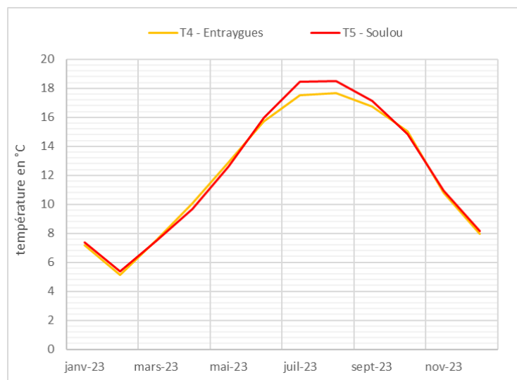
Figure 3 : Températures moyennes mensuelles du Lot à l'aval du barrage de Castelnau et à l'aval de la confluence avec la Truyère
