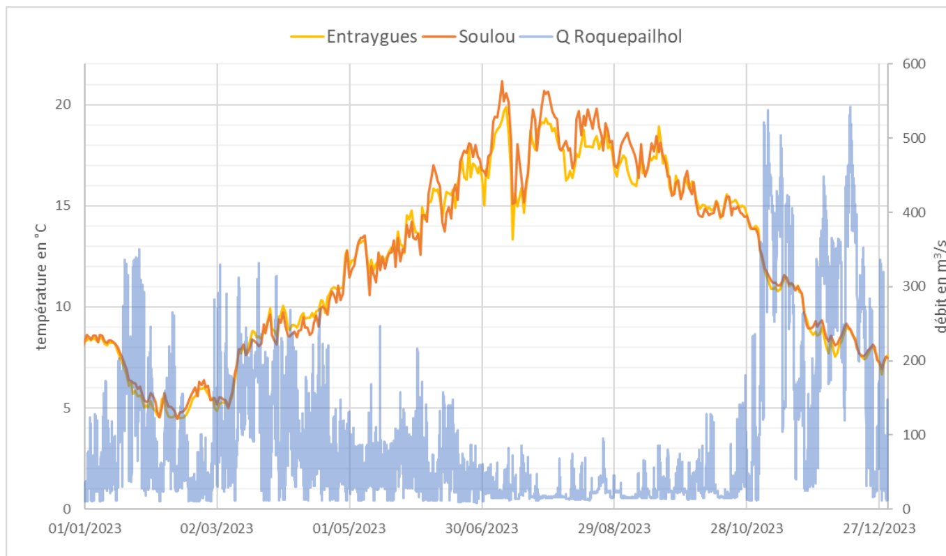
Figure 7 : Régime thermique moyen journalier du Lot à l'aval de la confluence avec la Truyère – T4 et T5 de janvier à décembre 2023
