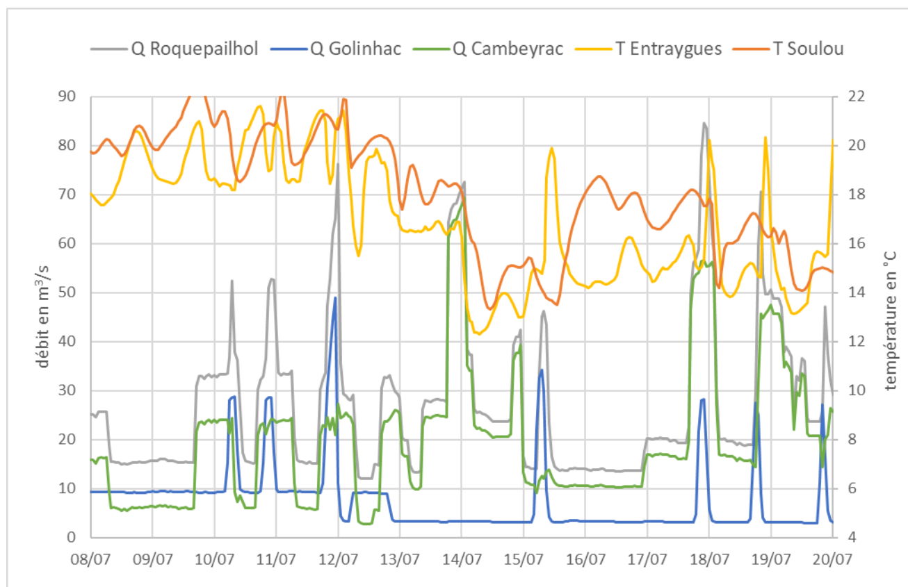
Figure 9 : Influence de l'hydrologie sur le régime thermique instantané du Lot à l'aval de la confluence avec la Truyère en juillet 2023
