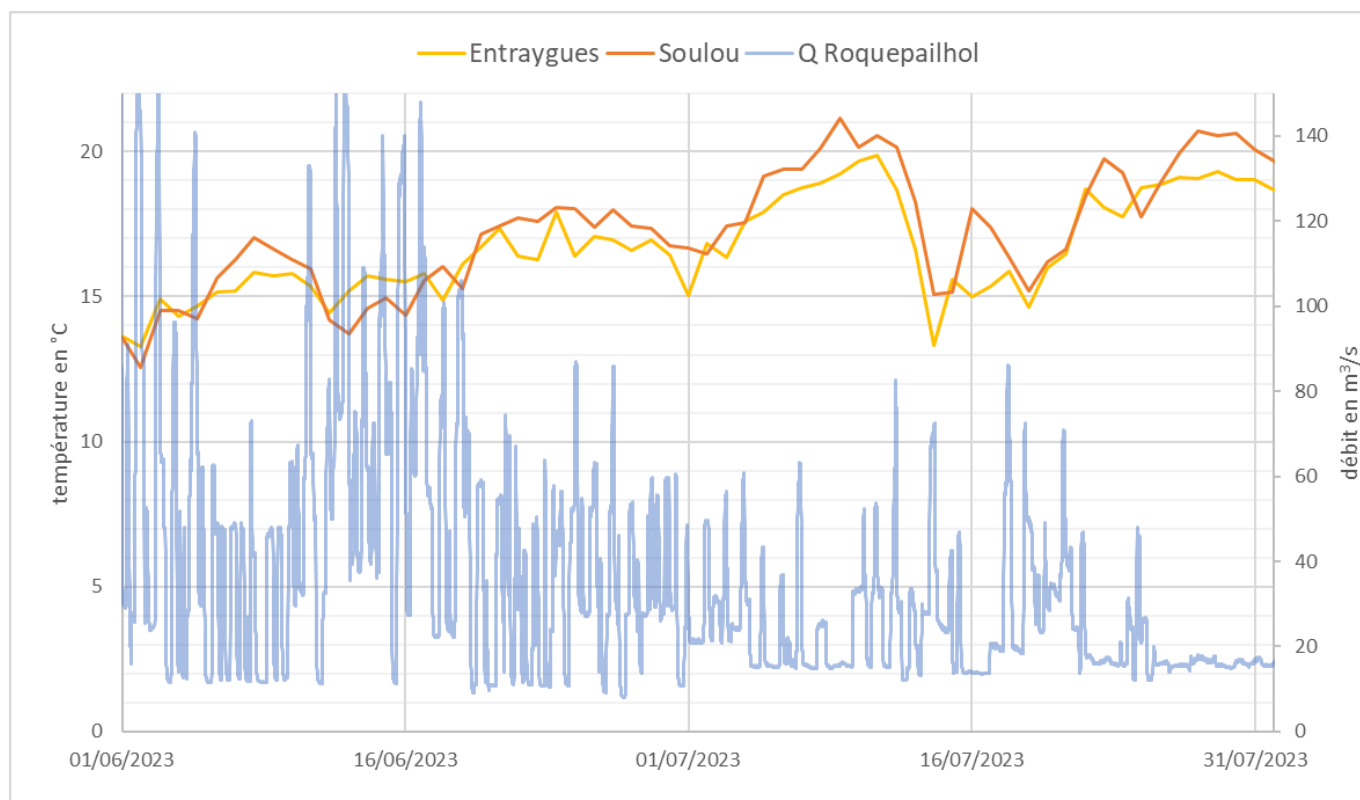
Figure 8 : Régime thermique moyen journalier du Lot à l'aval de la confluence avec la Truyère en juin et juillet 2023
