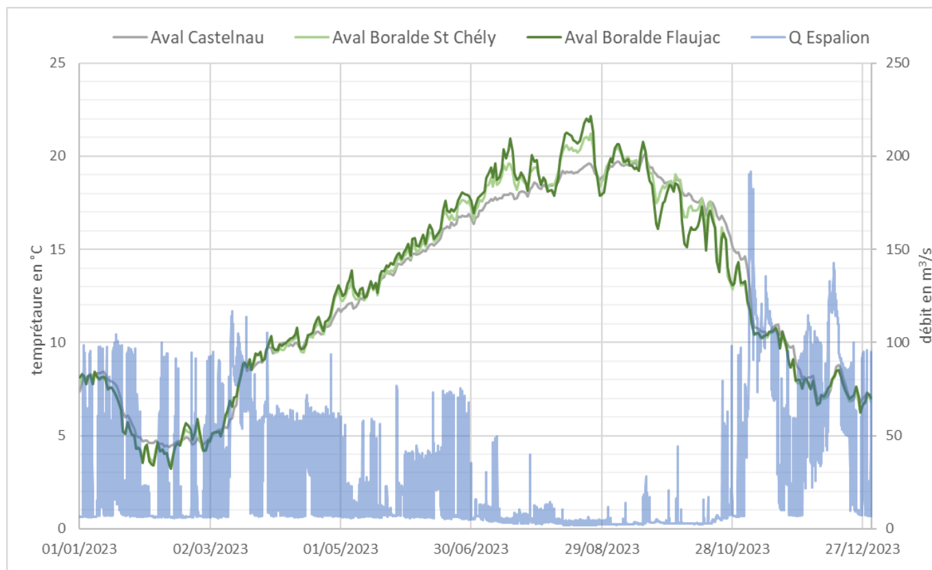
Figure 6 : Régime thermique moyen journalier du Lot à l'aval de Castelnau – T1, T2 et T3 de janvier à décembre 2023
