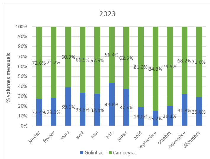
Figure 5 : Proportions des volumes issus de la branche Truyère et de la branche Lot, sur le Lot à Roquepailhol en 2023
