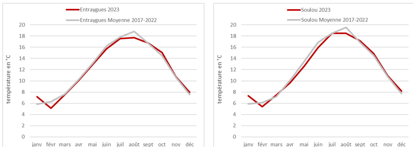
Figure 4 : Comparaison des températures moyennes mensuelles du Lot de T1 à T5 au cours de l'année 2023 avec les températures moyennes mensuelles interannuelles (2017-2022 ou 2018-2022 selon les stations)
